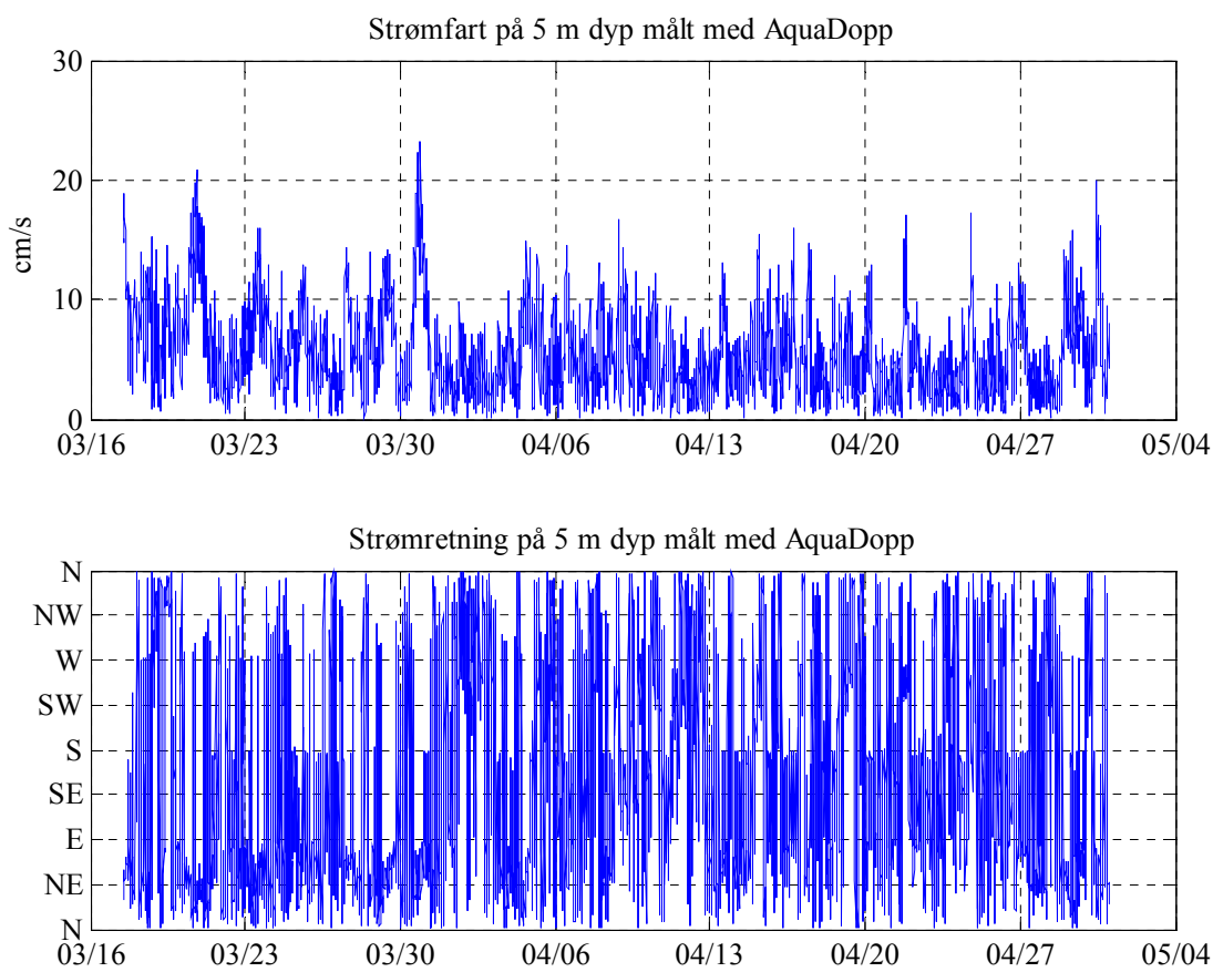
Fig. 14. Strømfart og retning i perioden 17. mars-30.april 2008.
